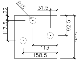
MODULO B
