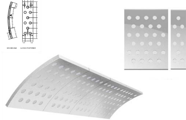
PIEZA TIPO D + D1
