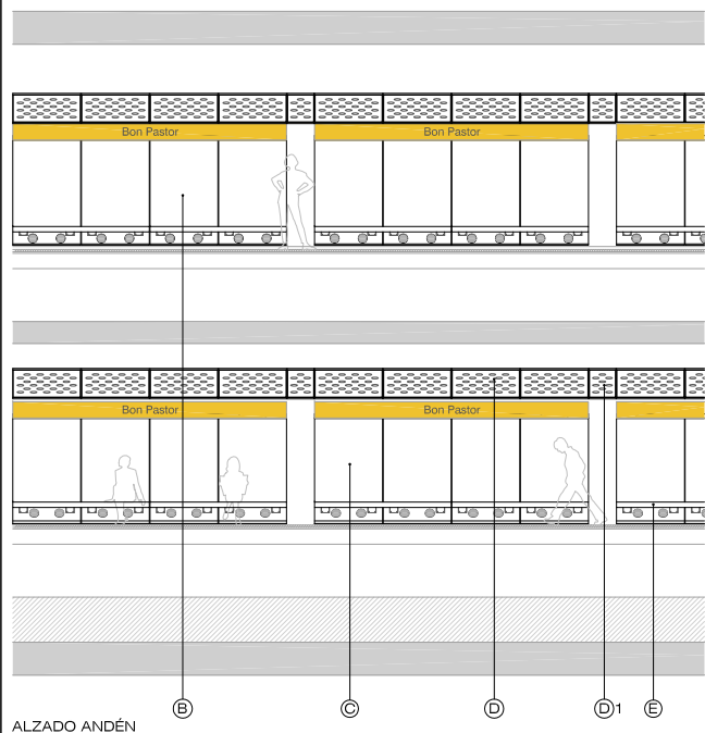
ALZADO ANDÉN
