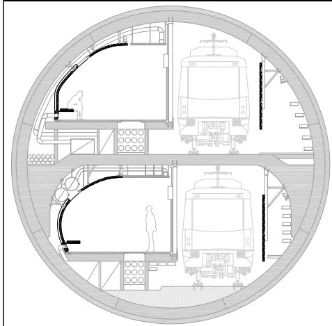
SECCIÓN
