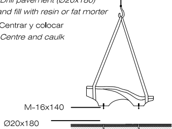
MODULOS B y C ANCLADOS ANCHORED B and C MODULES
