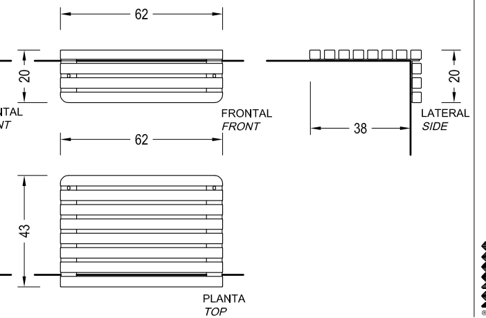
D. UNIVERSE asiento / seat
