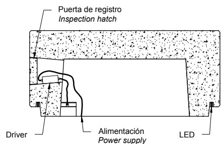
SECCIÓN REGISTRO ELECTRICAL BOX SECTION
