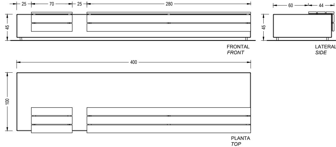
LONGO BANCA + ACCESORIO BANCA + ACCESORIO ASIENTO (2730 kg)
