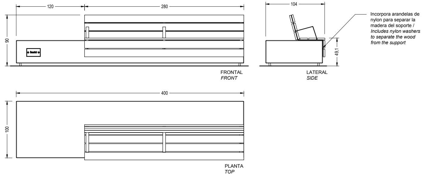
LONGO BANCA LED + ACCESORIO BANCO (2758 kg)
