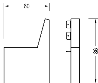
Soporte Banca Doble 95 kg Ref. ALPINE-BCO-CNT
