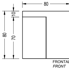
PRAT mesa / table
