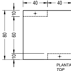
PRAT-MINI mesa / table
