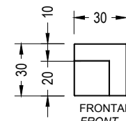
PRAT-MINI taburete / stool
