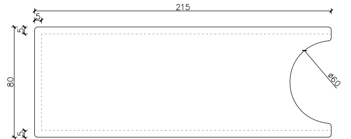
PLANTA
