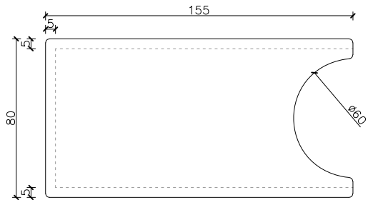
PLANTA
