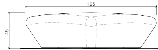
FRONTAL
