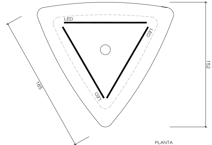
PLANTA
