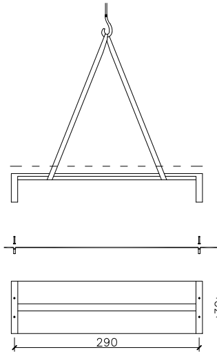
elevación / hoisting (P=537 kg)
