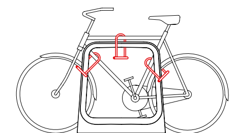
Aparcamiento de bicicletas con tres puntos de unión mediante candados de uso común
