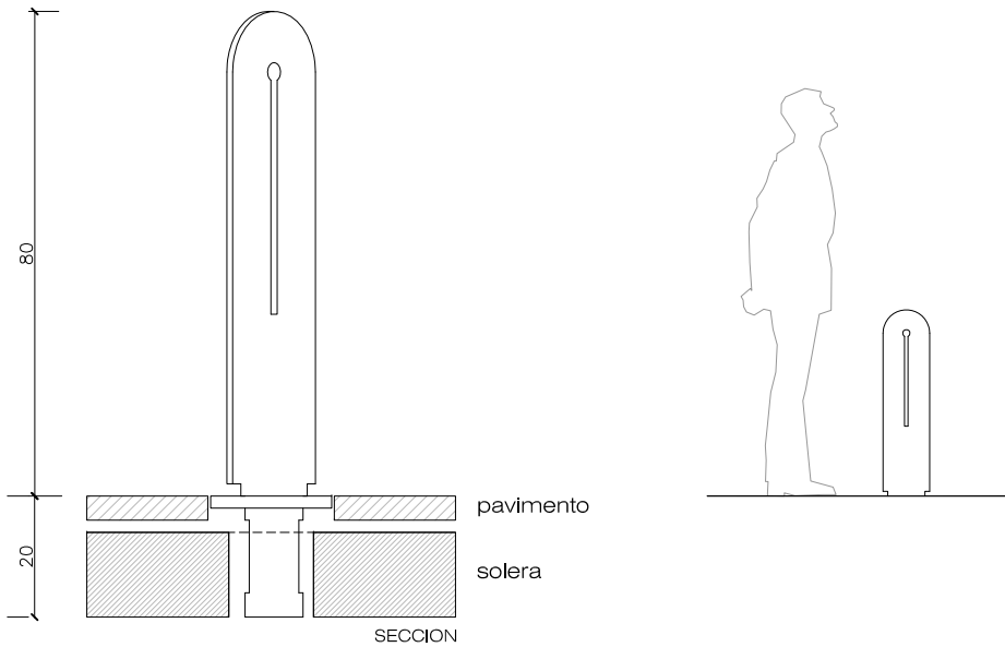
EJEMPLO DE COLOCACIÓN EN PAVIMENTO DE PANOT 20x20
