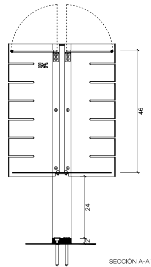
SECCIÓN A-A'
