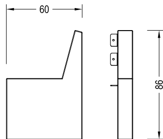
Soporte Banco Doble 95 kg Ref. ALPINE-BCO-CNT
