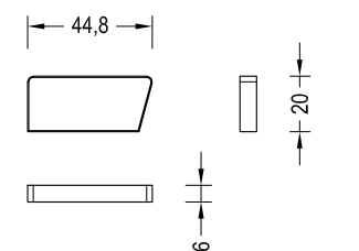
Accesorio Apoyabrazos 2,3 kg Ref. ALPINE-APOY-ACC
