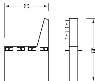
Soporte Banca-Banco 95 kg Ref. ALPINE-BCA-BCO
