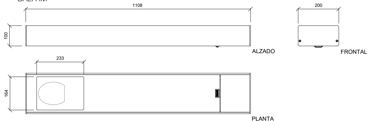
BALI HM
