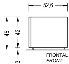
BOX RADIUS 45°
