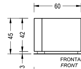
BOX RADIUS 90°
