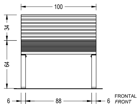
LASAI chaise-longue 100
