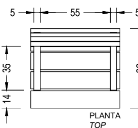
ACCESORIO ASIENTO
