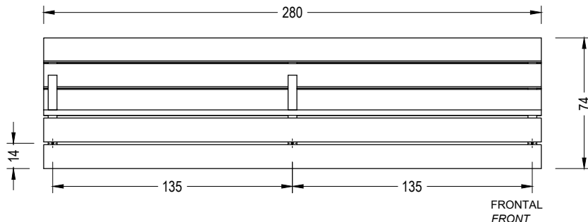
ACCESORIO BANCO
