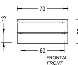
ACCESORIO ASIENTO
