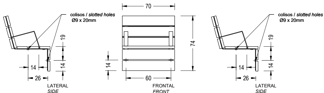
ACCESORIO SILLA
