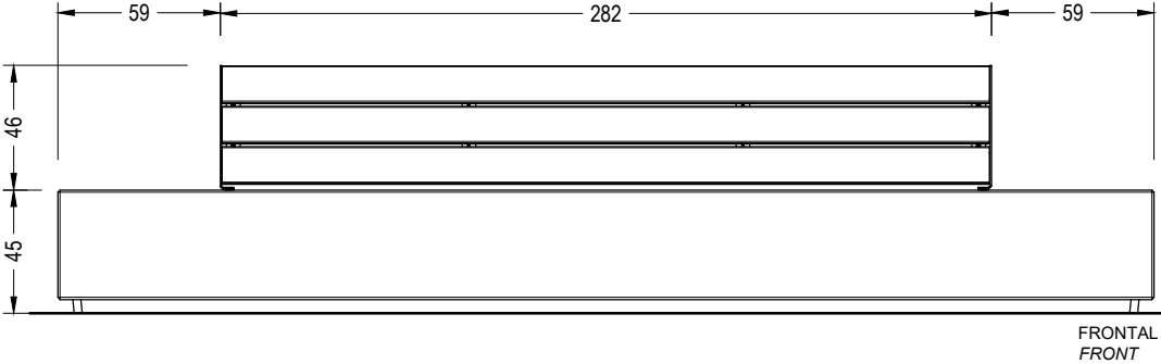
LONGO BANCA + ACCESORIO RESPALDO DOBLE (2730 kg)
