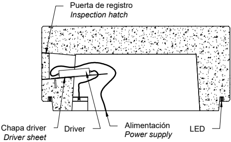
SECCIÓN REGISTRO ELECTRICAL BOX SECTION
