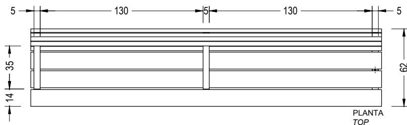
ACCESORIO BANCA
