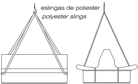
BANCO APOYADO SIN ANCLAJE FREE-STANDING BENCH
