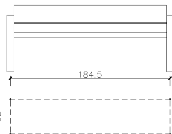
elevación / hoisting (P= 85 Kg.)
