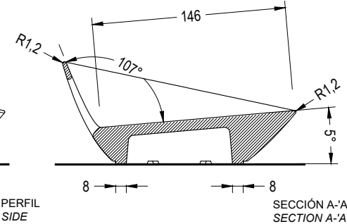
SECCIÓN A-A SECTION A-A
