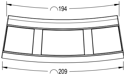
PLANTA INFERIOR BOTTOM PLAN
