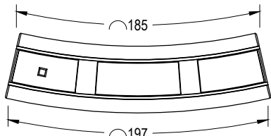
PLANTA INFERIOR BOTTOM PLAN
