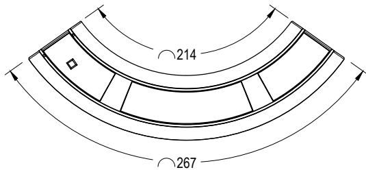
PLANTA INFERIOR BOTTOM PLAN
