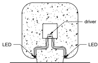
SECCIÓN REGISTRO ELECTRICAL BOX SECTION
