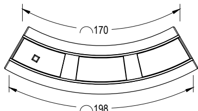
PLANTA INFERIOR BOTTOM PLAN
