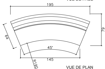
VUE DE PLAN
