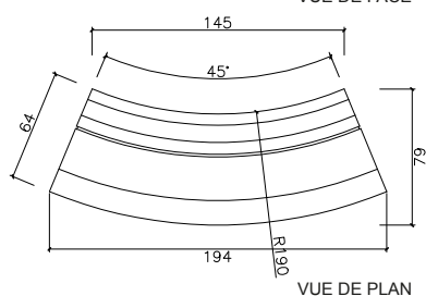
VUE DE PLAN
